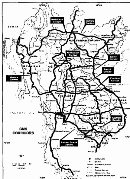
รูปที่ ๑ อนุภูมิภาคลุ่มน้ำโขง (ที่มา ADB, CIA, Wikipedia)
